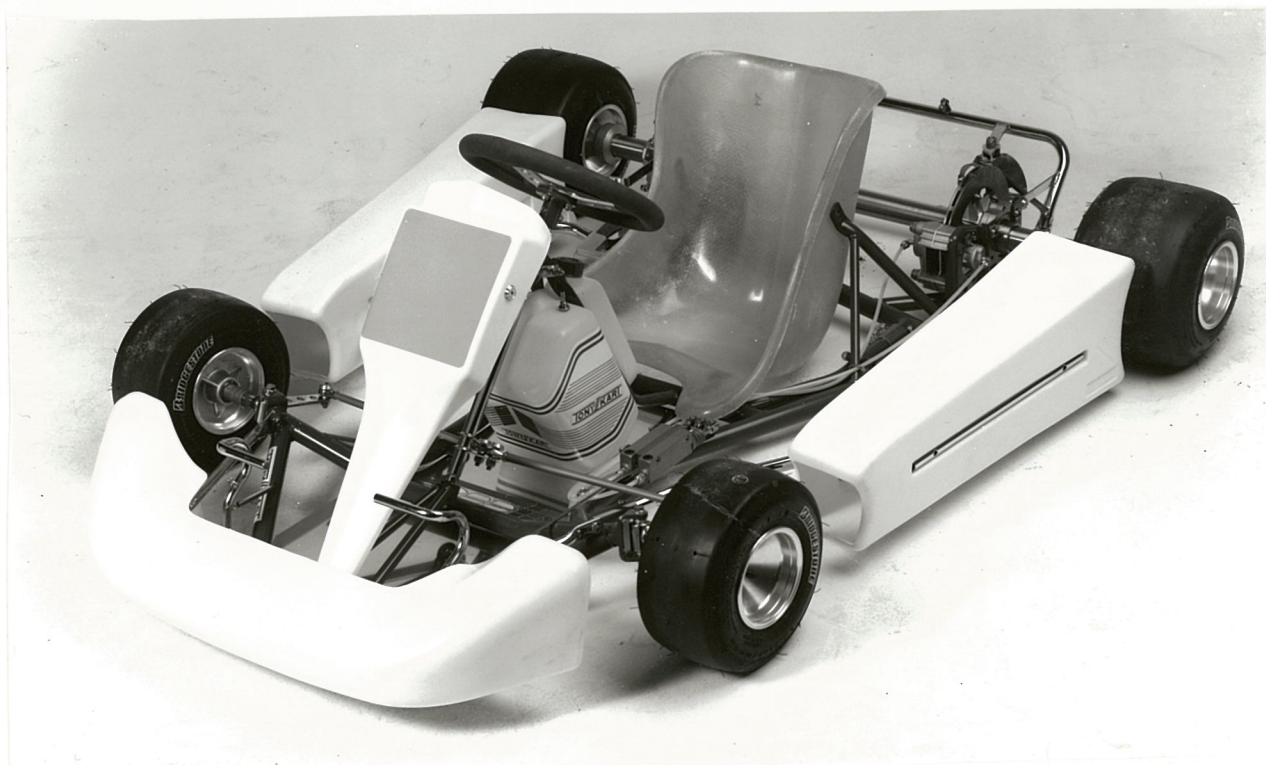
Photo du châssis avec pneumatique
